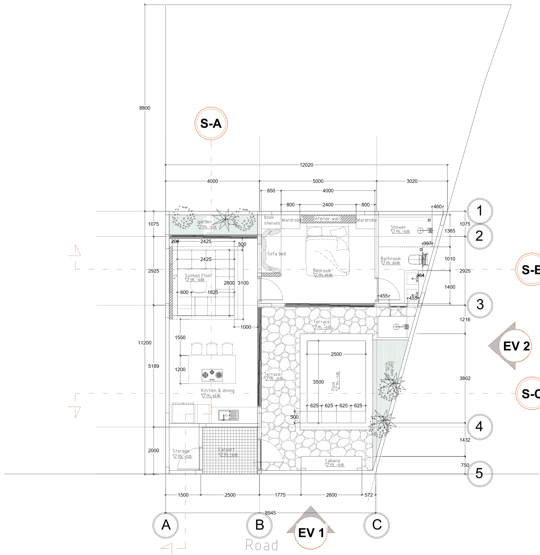
Layout Plan Skala 1:100
